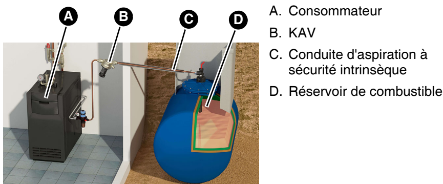
Figure 5: Montage avec conduite d'aspiration à sécurité intrinsèque
