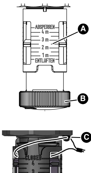
Abbildung 8: Plombierung befestigen
