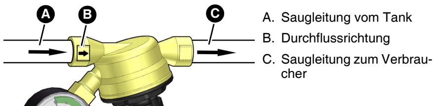
Abbildung 4: Montage
