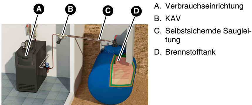
Abbildung 5: Montage mit selbstsichernder Saugleitung
