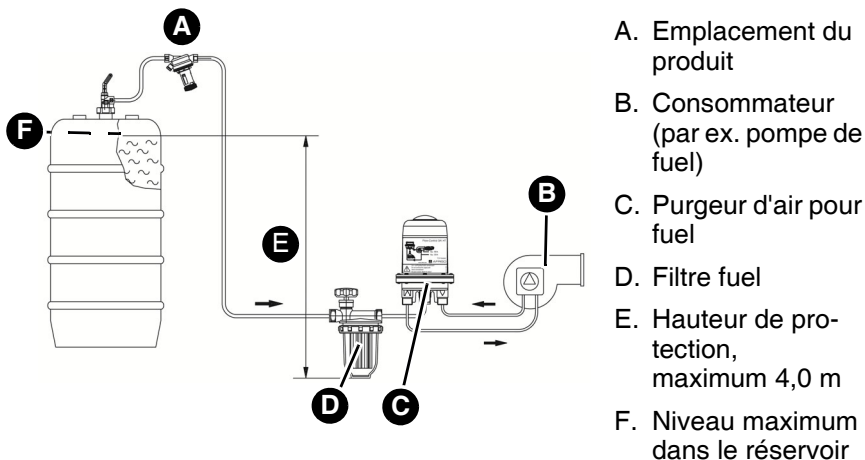
Figure 7: Hauteur de protection = différence de hauteur entre le niveau maximum dans le réservoir et le point le plus bas de la conduite d'alimentation
