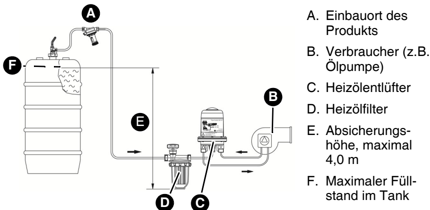
Abbildung 7: Absicherungshöhe = Höhendifferenz zwischen maximalem Füllstand im Tank und tiefstem Punkt der Zuleitung
